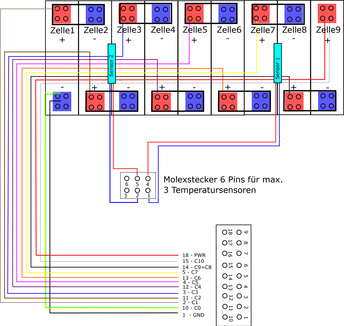
Molexstecker 18 Pins
