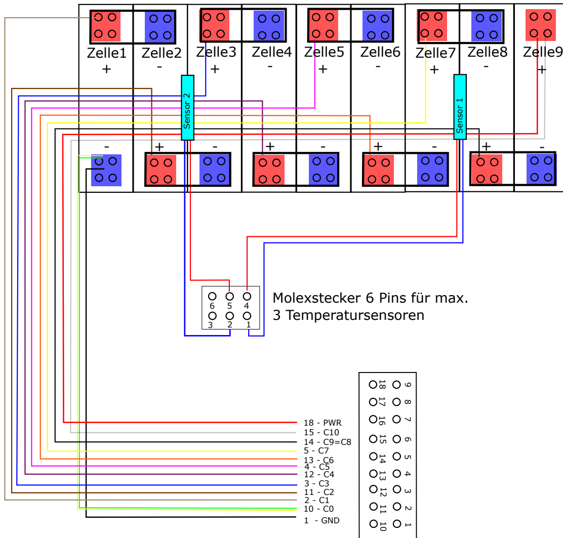
Molexstecker 18 Pins
